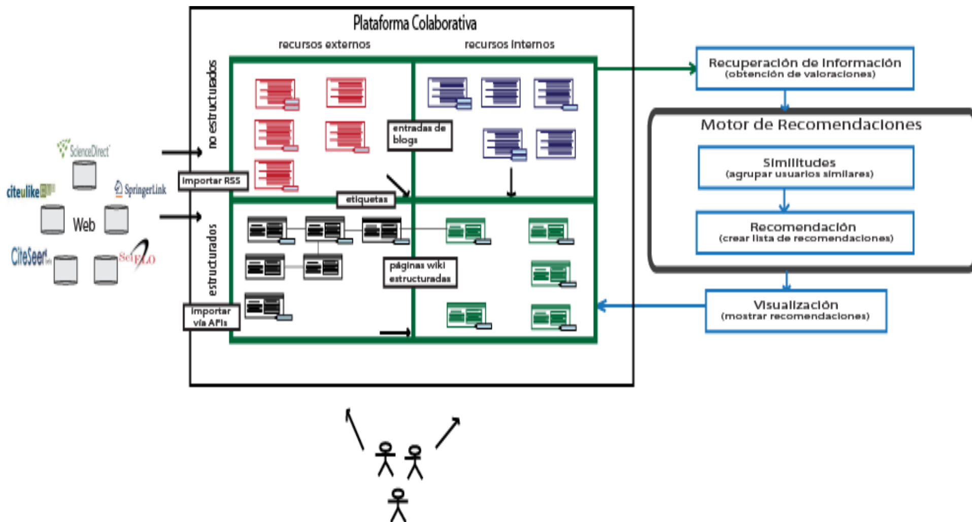
Figura 1. Modelo de vigilancia tecnológica apoyada por un sistema de recomendaciones basado en el filtrado colaborativo.
