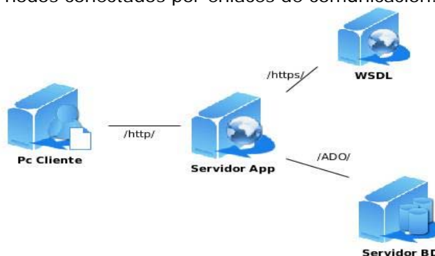
Figura 4. Diagrama de Despliegue de la Aplicación
