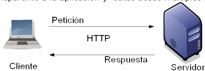
Figura 2. Cliente-Servidor
